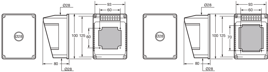
Caja 16A / 16A Box
