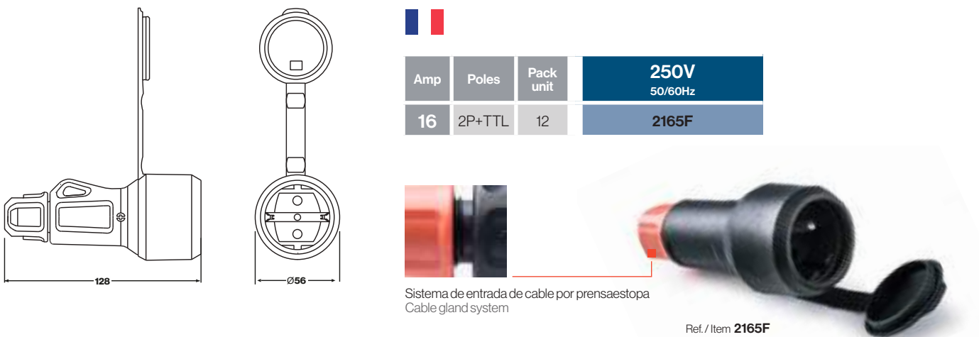
Base móvil 2P+T 16A 250V FR desmontable IP54 / Mobile socket 2P+T 16A 250V FR detachable IP54 - Ref.Item 2165F
