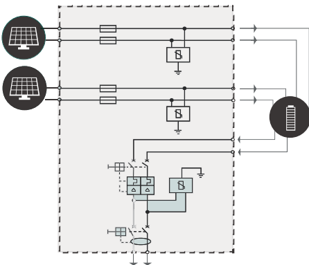
*Esquema Ref. E3SBAC08-FVC110 *Ref. E3SBAC08-FVC110 diagram
