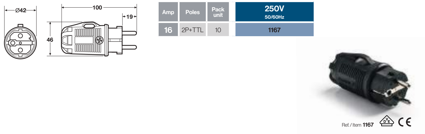
Clavija de goma IP54 / Rubber plug IP54 - Ref.Item 1167
