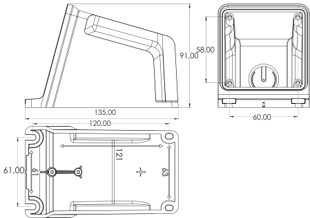
Caja 16/32A / Box 16/32A
