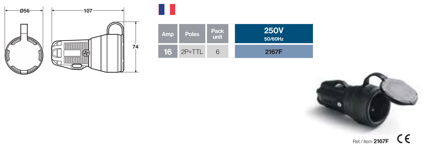
Base de goma IP54 / Rubber socket IP54 - Ref.Item 2167F
