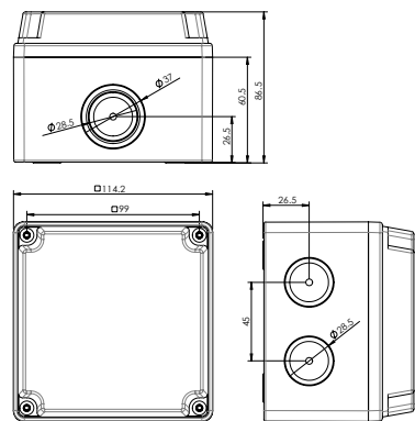
Caja de conexión 1 toma / Junction box for 1 socket Ref. Item 23021
