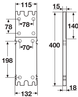
Placa modular para tomas de corriente interblocantes / Modular plate for interlocked sockets Ref. Item 23023
