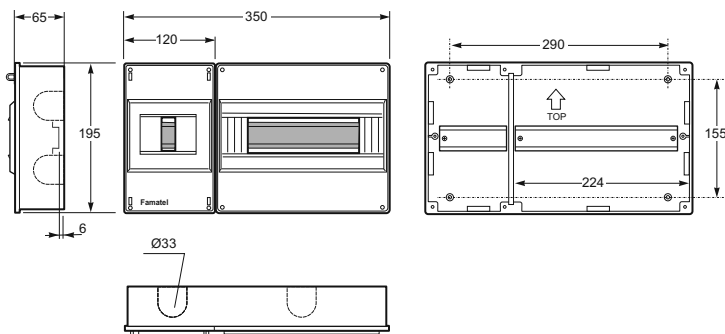
Cajas modulares de superficie ICP / ICP Surface boxes - Ref. Item 3413
