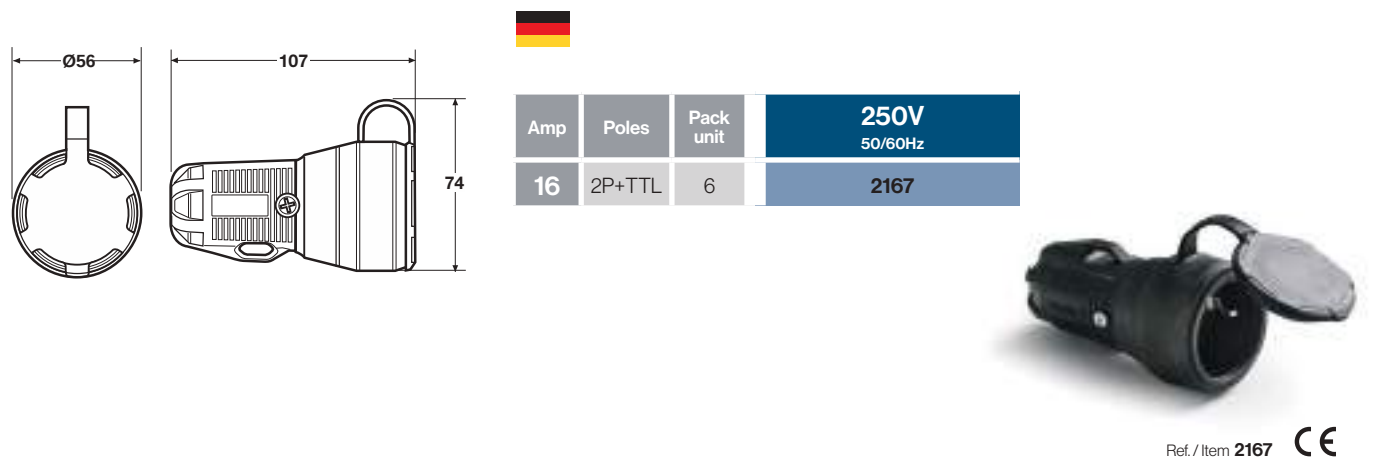
Base de goma IP54 / Rubber socket IP54 - Ref.Item 2167F
