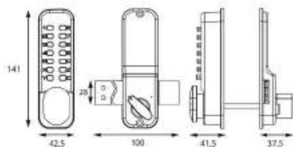
MCA200
