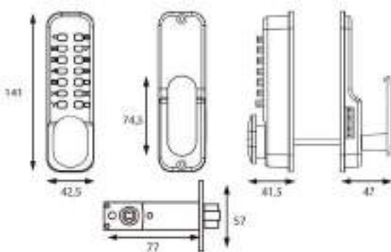
MCA100
