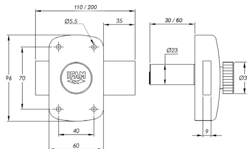
Cod. 900820 Cod. 901020 Cod. 901270 Cod. 901570 PAG. 95
