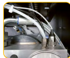
Regulador de aspiración Sistema electro-neumático normalmente abierto. Regula el funcionamiento del compresor garantizando la mínima presión necesaria durante la marcha en vacío para lograr el máximo ahorro energético
